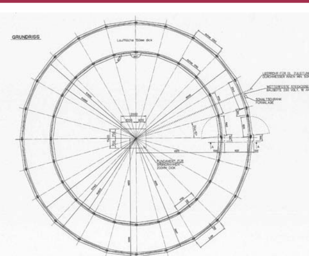
Giostra per cavalli con elemento di recinzione, pianta di base
